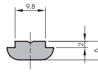
Nutenstein einschwenkbar
