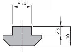
Nutenstein einschiebbar
