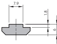
Nutenstein einschiebbar
