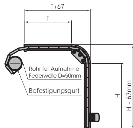
Schnitt A-A
