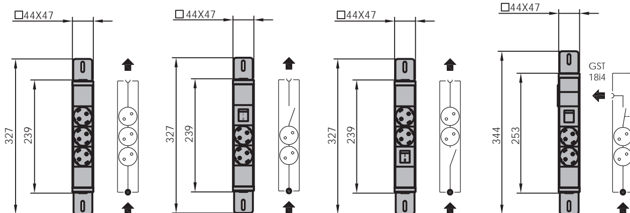
Steckdosenleiste 3S
